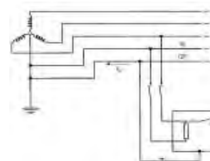
Figura 3. Esquema TN-S.
