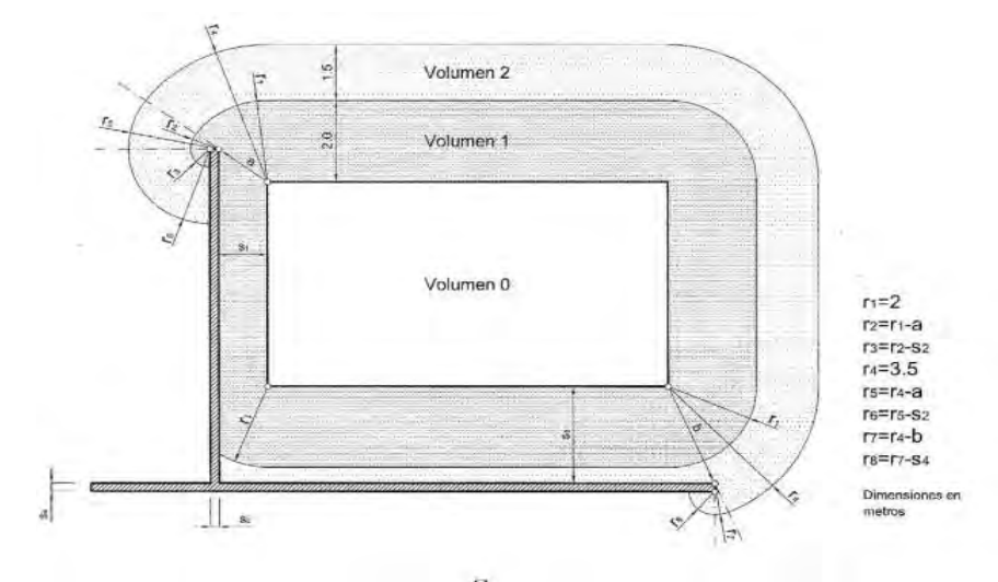
Figura 4. Volúmenes de protección en piscinas con paredes
