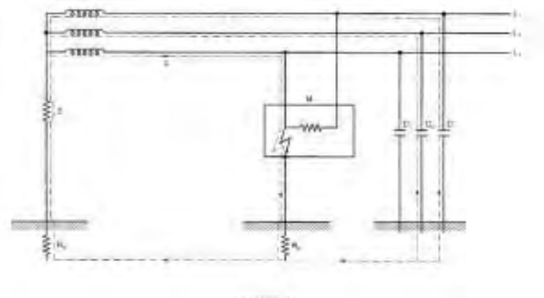
Figura 6. Esquema IT unido a tierra por impedancia Z y con las puestas a tierra de la alimentación y de las masas separadas
