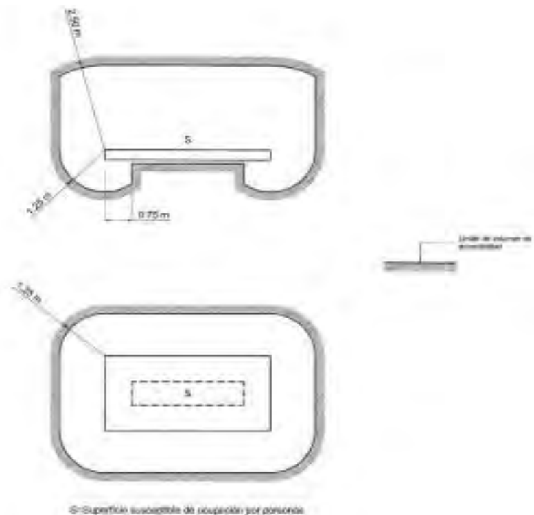
Figura 1. – Volumen de accesibilidad
