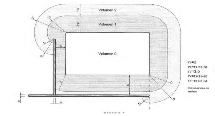
Figura 4. Volúmenes de protección en piscinas con paredes
