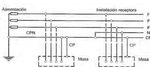
Figura 3. Esquema de distribución tipo TN-C-S
