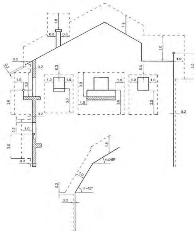
Figura 1. Zona de protección en edificios para la instalación de líneas eléctricas de baja tensión con conductores desnudos.
