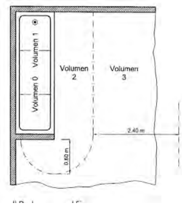
Figura 2 – BAÑERA CON PARED FIJA
