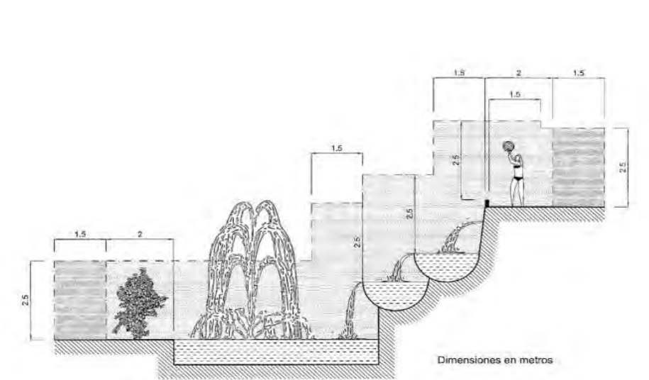
Figura 5. Volúmenes de protección en fuentes
