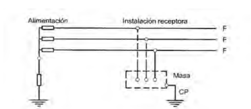
Figura 5. Esquema de distribución tipo IT
