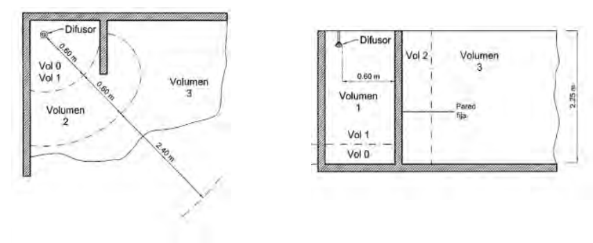
Figura 6 – DUCHA SIN PLATO PERO CON PARED FIJA. DIFUSOR FIJO
