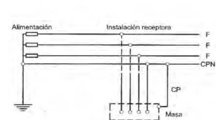
Figura 2. Esquema de distribución tipo TN-C
